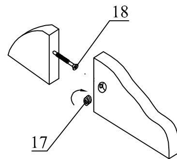
Рис.5 Крепление деталей эксцентриком
